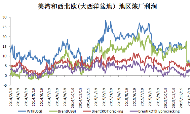
图 3：炼油利润
