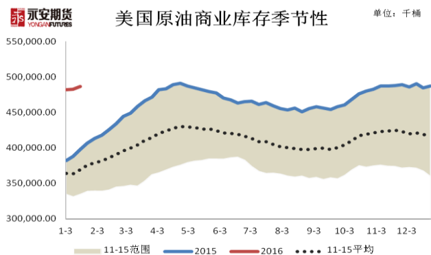
图 4：EIA 报告
