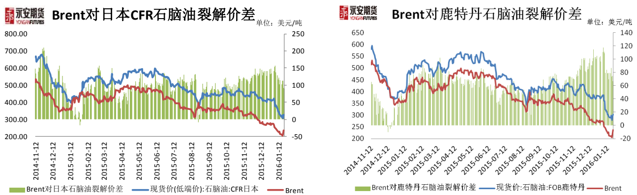
图 2：裂解价差
