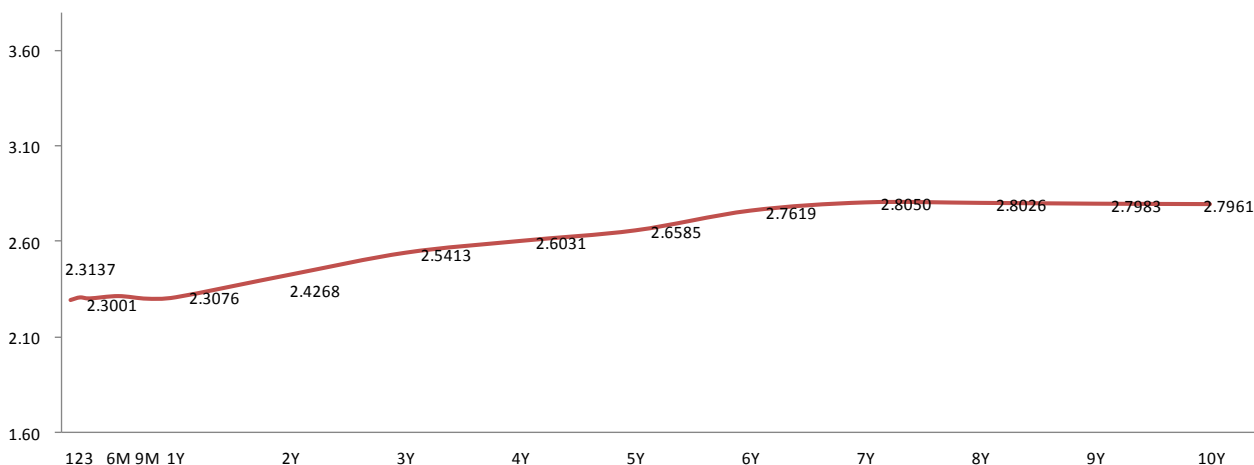
图 5：国债到期收益率曲线（2015-12-28）
